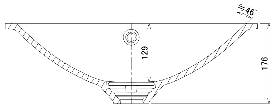
A-A 断面図
