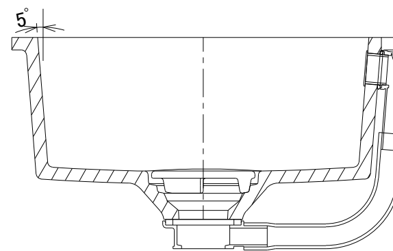
B-B 断面図
