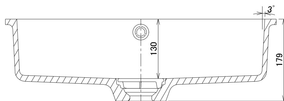
A-A 断面図
