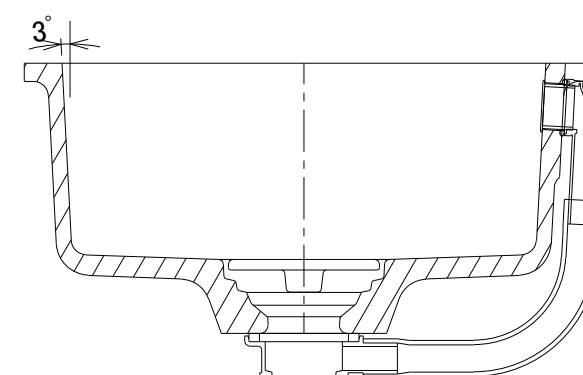
B-B 断面図
