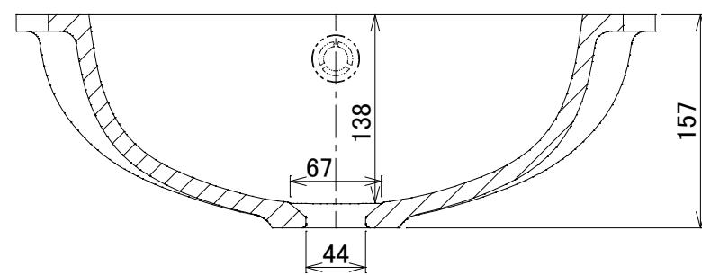
A-A 断面図
