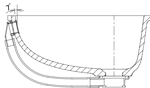
B-B 断面図
