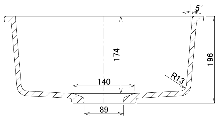
A-A 断面図
