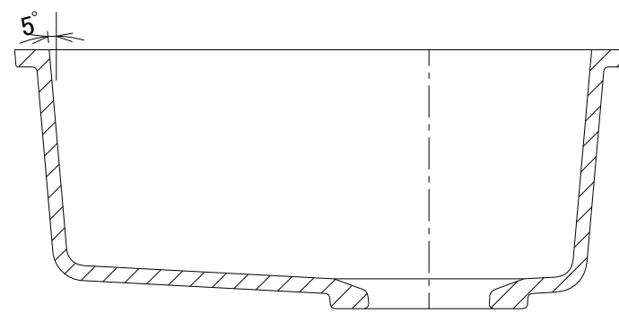
B-B 断面図
