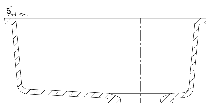
B-B 断面図
