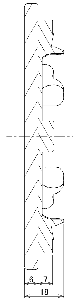
A-A 断面図
